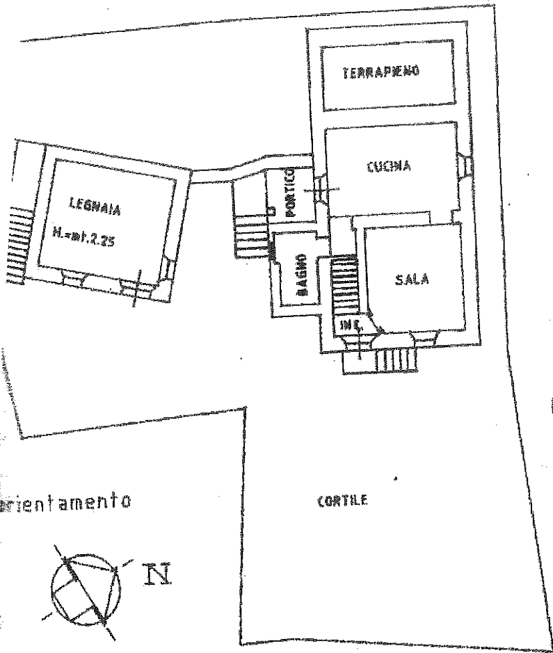
PIANO TERRA - H. = mt. 2.05
